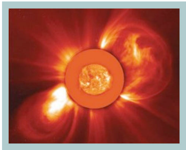
Figura 4. En esta imagen se muestran 2 EMC simétricamente opuestas. Las observaciones se realizaron el 8.Diciembre.2000 con la nave espacial SOHO, utilizando el coronógrafo LASCO-C2. Una imagen del EIT tomada el mismo día ha sido superpuesta en lo que sería el coronógrafo C2, el cual es usado para ocultar la luz fotosférica y poner así de manifiesto la débil señal coronal en luz blanca. ( Solar & Heliospheric Observatory, SOHO ).
