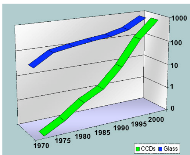
Figura 1. La gráfica muestra el crecimiento de los espejos primarios de los telescopios y de las dimensiones de los detectores CCD respecto al tiempo. Claramente se puede ver que el aumento de la resolución de los CCDs cumple con la ley de Moore, es decir, presenta un crecimiento exponencial.
